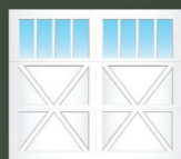
IX04S
