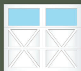
IX01S
