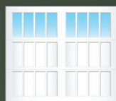
I304S
