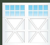
IX08S
