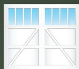
IA04S
