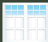
I106S
