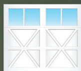
IX02S
