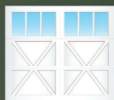
IX03S
