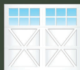
IX06S
